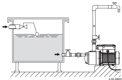
Fig. 1 Funzionamento sotto battente Positive stion head operation Zulaufbetrieb Fonctionnement en charge Funcionamiento bajo carga Tilrinning sugsidan Toeloopsituatie Θέση λειτουργίας με θετική αναρρόφηση Работа под гидравлическим напором 正吸上水头的操作
